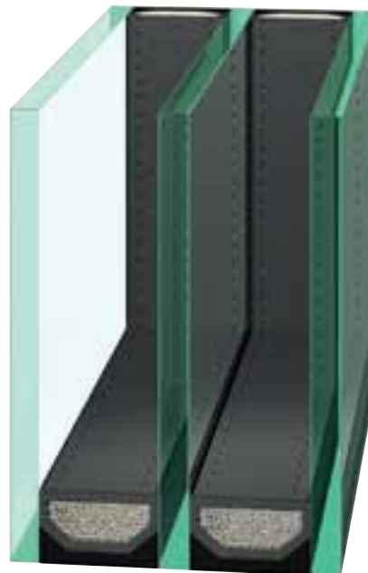
3-fach-Energiesparglas
