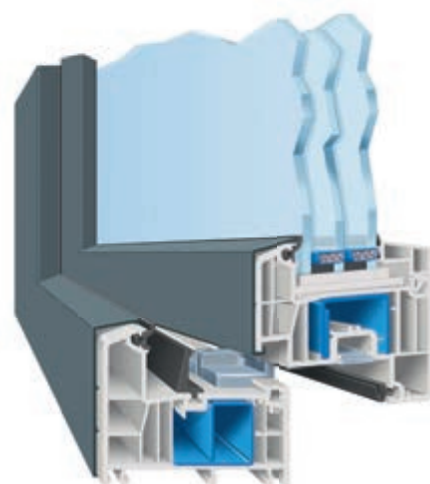
AFINO-top MD (Mitteldichtungssystem mit drei Dichtungen)
