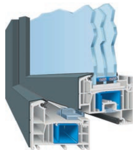
AFINO-top AD (Anschlagdichtungssystem mit zwei Dichtungen)
