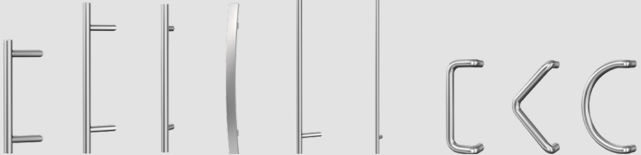
Außengriff G101sf-E, Länge 400 mm Außengriff G102sf-E, Länge 600 mm Außengriff G102gf-E, Länge 600 mm Außengriff G112gf-E, Länge 600 mm Außengriff G103sf-E, Länge 1.000 mm Außengriff G104gf-E, Länge 1.500 mm Außengriff G006gf-E, Länge 330 mm Außengriff G007gf-E, Länge 330 mm Außengriff G009gf-E, Länge 330 mm
